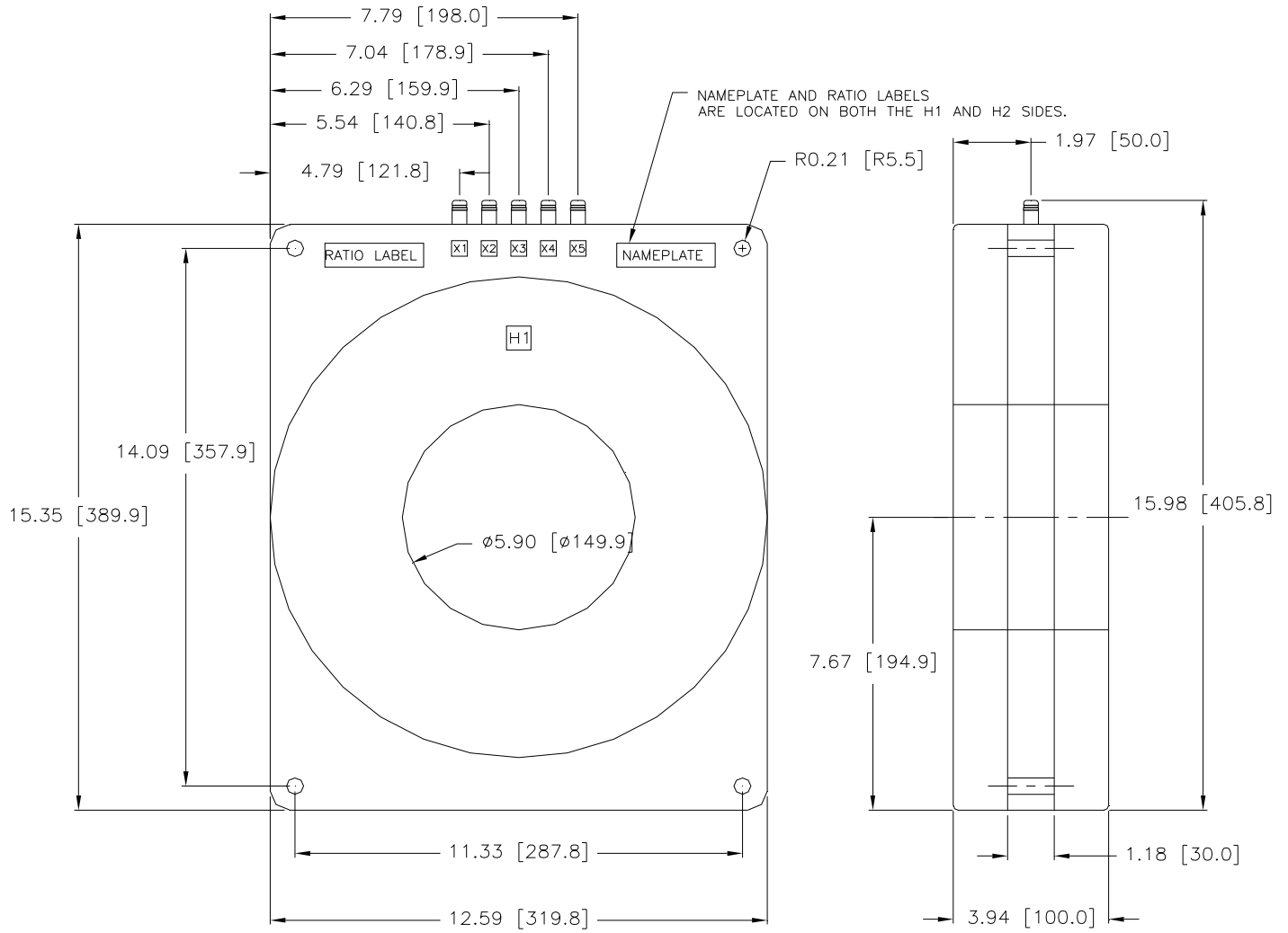
ANSI 600:5 TAPS
