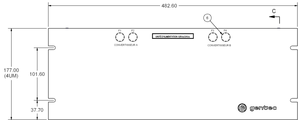
VUE AVANT
