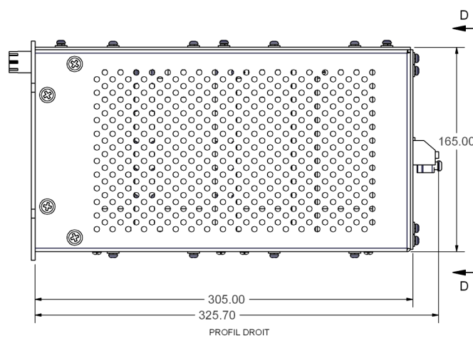
PROFIL DROIT
