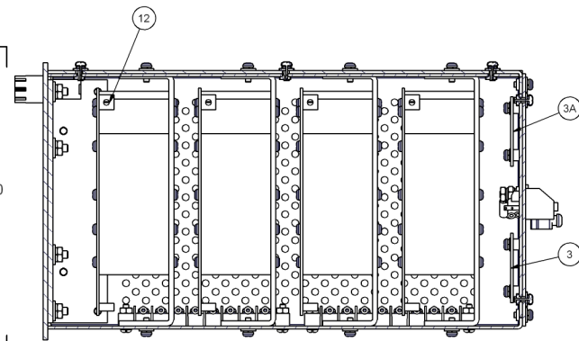
COUPE C-C
