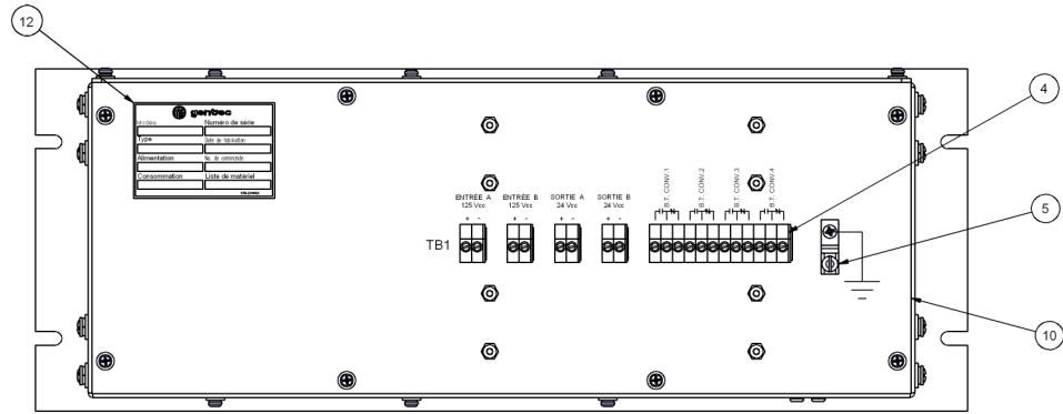
VUE ARRIÈRE
